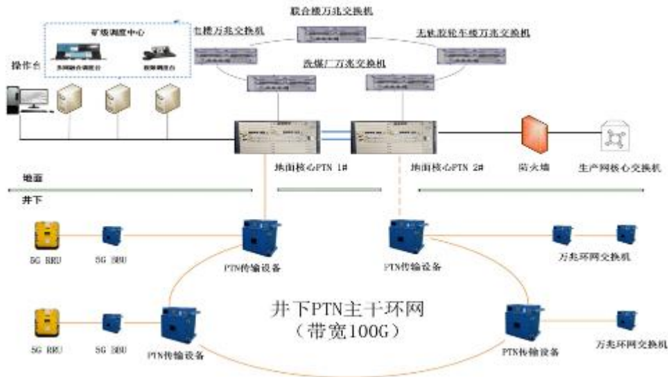
图：测试床井下融合组网应用方案
