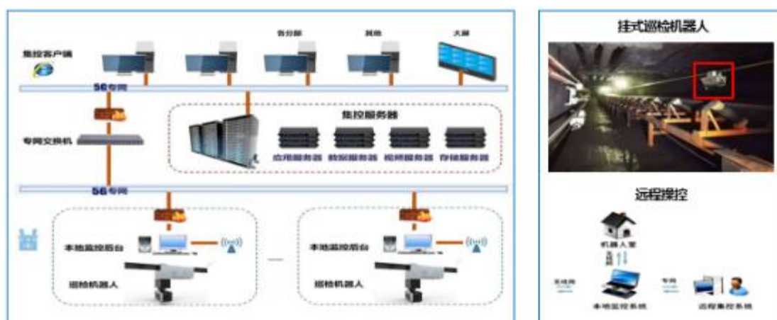
图：测试床5G机器人巡检应用方案
